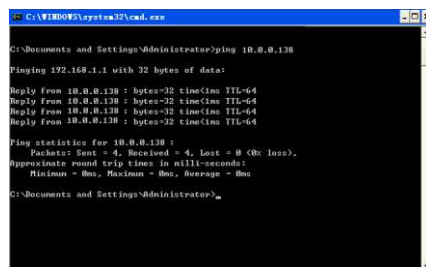
Obrázek 5 Příkaz Ping
